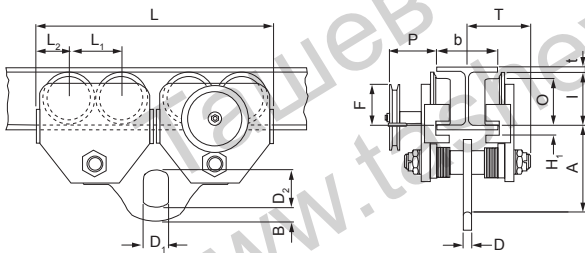
HTG, 15000 - 20000 kg
