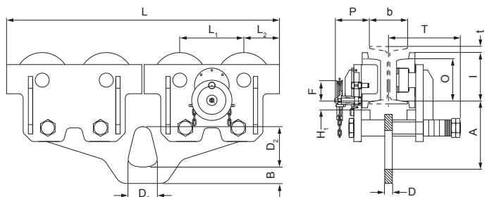
HTG, 50000 kg
