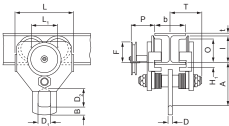
HTG, 10000 kg
