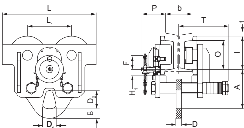
HTG, 30000 kg
